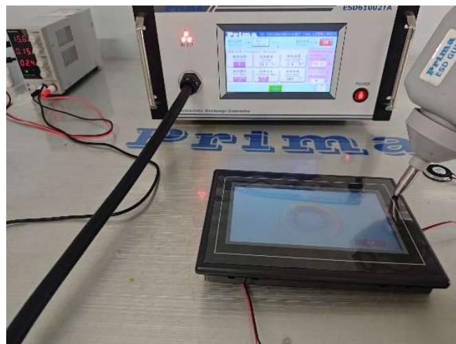
图 5-2 ESD 测试图
