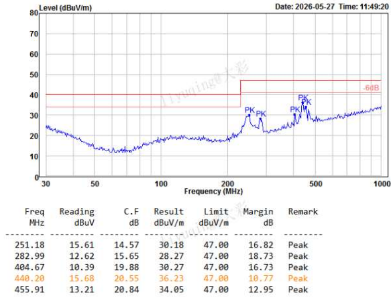
图 5-6 RE 测试水平方向
