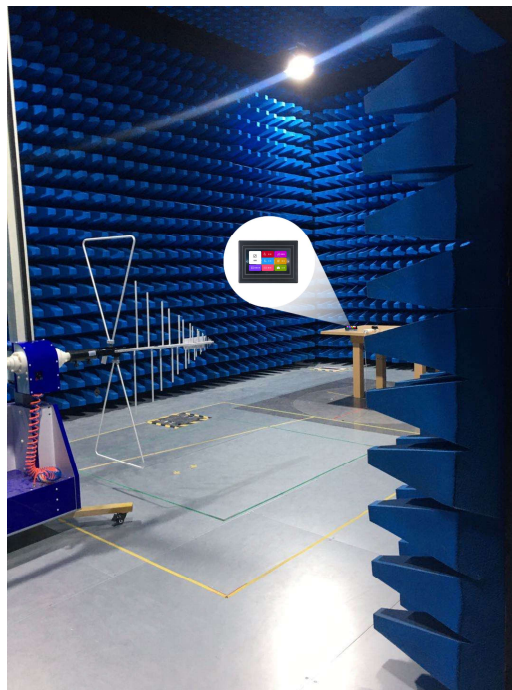
图 5-5 RE 测试图
