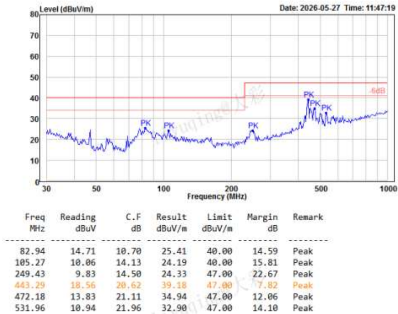
图 5-7 RE 测试垂直方向
